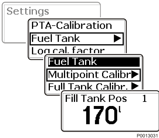
Калибровка топливной цистерны по нескольким точкам
