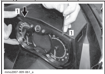
1. Защелка
