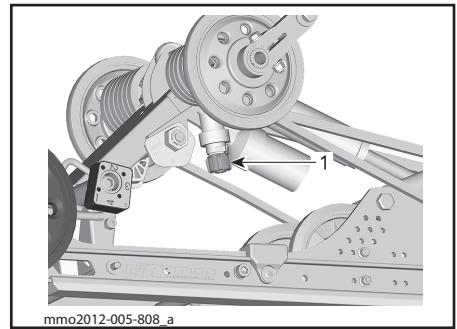
1. Регулятор силы демпфирования сжатия
