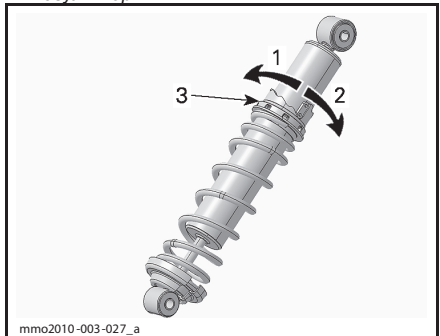
ТИП РЕГУЛЯТОРА - АМОРТИЗАТОР С ГАЗОВЫМ ПОДПОРОМ ВЫСОКОГО ДАВЛЕНИЯ (HFG)
