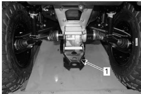
1. Задняя буксировочная проушина
