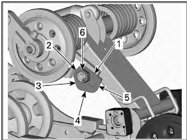
ПОДВЕСКА rMOTION БЕЗ ВЫНОСНЫХ РЕГУЛИРОВОЧНЫХ ЭЛЕМЕН- ТОВ — ПОКАЗАНА ЛЕВАЯ СТОРОНА
