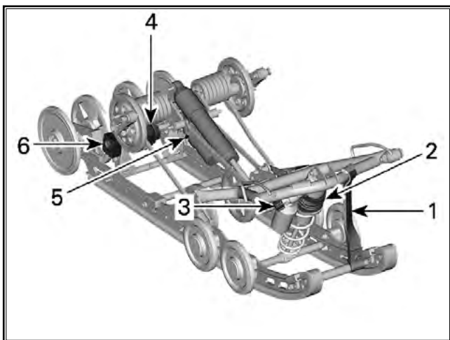
гMOTION БЕЗ ВЫНОСНЫХ РЕГУЛИРОВОЧНЫХ ЭЛЕМЕНТОВ — РЕГУЛИРУЕМЫЕ КОМПОНЕНТЫ
