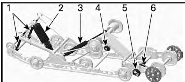
РЕГУЛИРУЕМЫЕ КОМПОНЕНТЫ SC5-U
