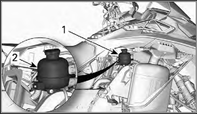
ТИПОВОЙ ВАРИАНТ 1. Расширительный бачок 2. Метка «COLD»
